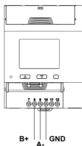
Fig. 11 Modbus RS485 (option S1)
